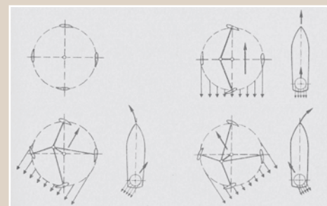
Schéma principu pohonu lodi pomocí naklápěcích lopatek v systému Voith Schneider Propeller
